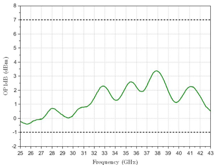
Figure 1: ERZ-LNA-2500-4300-33-2-NS P1dB
