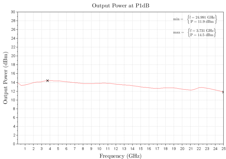
Figure 1: ERZ-LNA-0000-2500-14-2.5 P1dB
