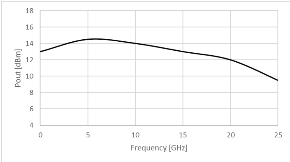
Figure 1: ERZ-LNA-0000-2500-14-2.5 P1dB
