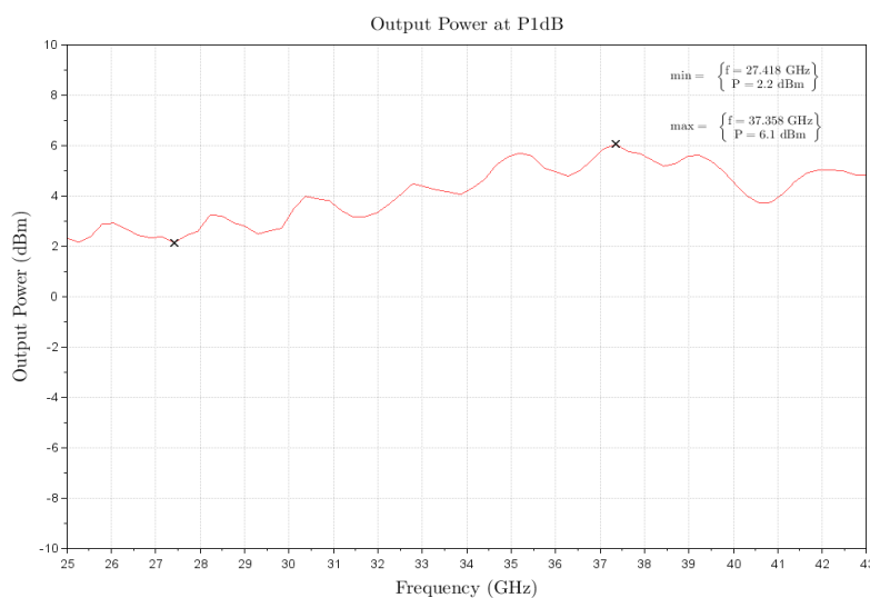
Figure 1: ERZ-LNA-2500-4300-33-2-NS P1dB
